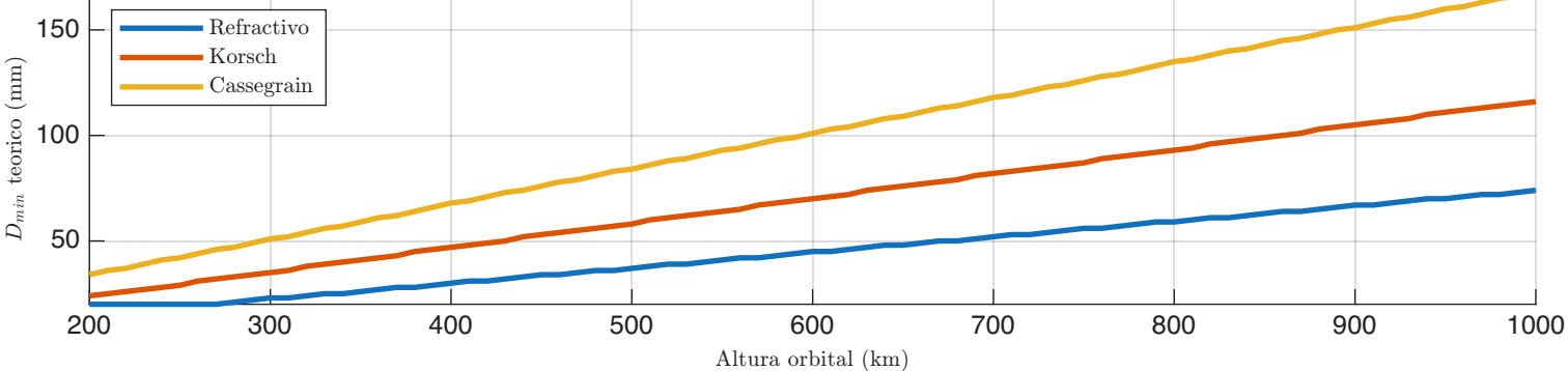
Detector 2: mínimo teórico por MTF/SNR - Configuración: 1 satélite(s), 2 telescopio(s) por satélite
